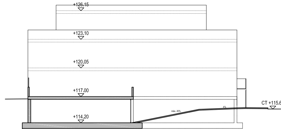
Alçat posterior
