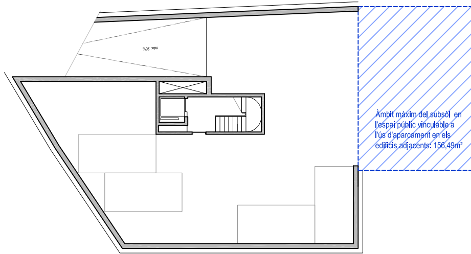
Planta soterrani
