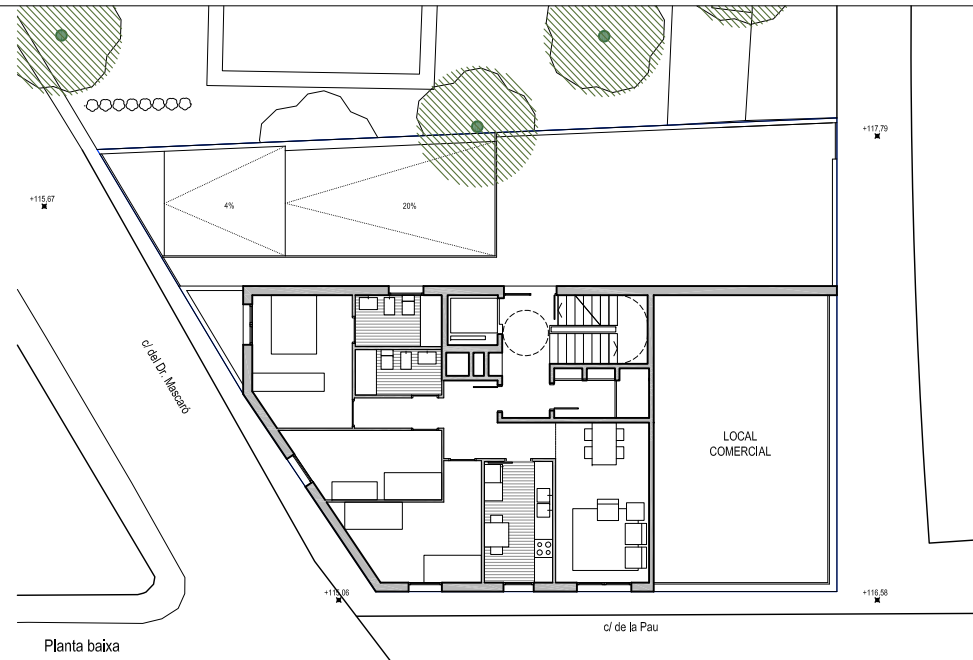
Planta baixa
