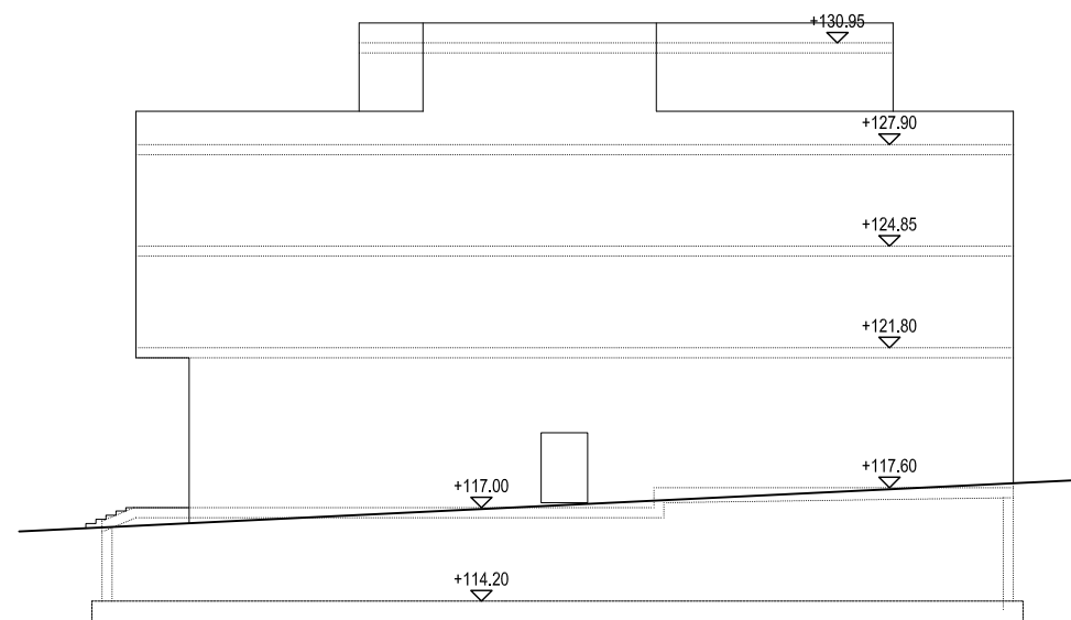
Alçat c/ Anselm Clavé
